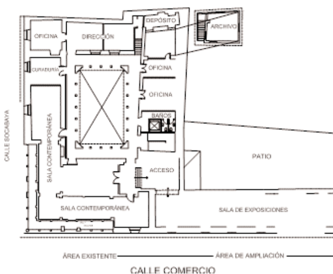
Segunda planta
