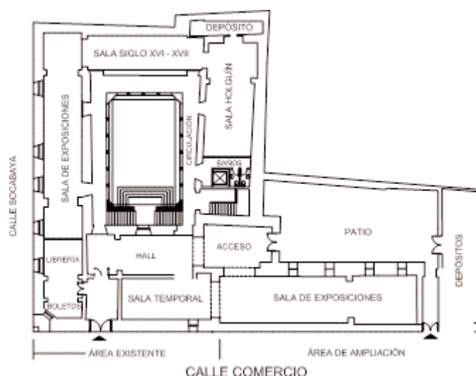
Primera planta
