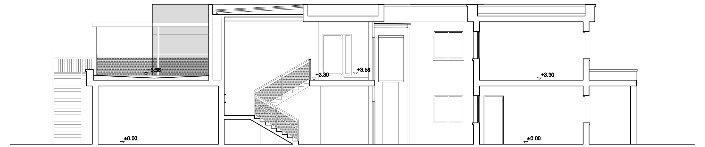
SECCION CC. ESTADO REFORMADO
