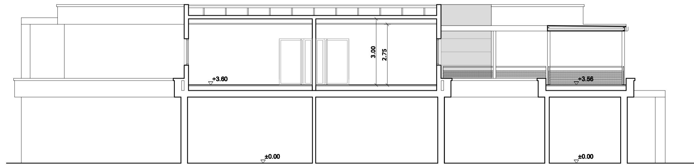
SECCION BB. ESTADO REFORMADO
