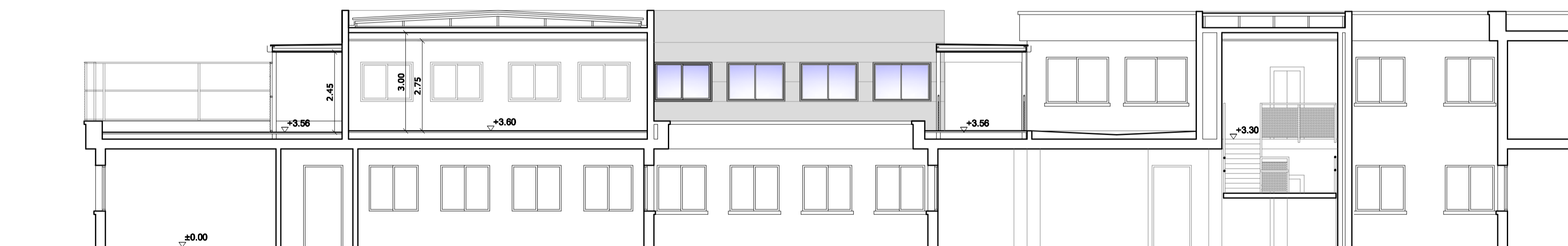
SECCION EE. ESTADO REFORMADO
