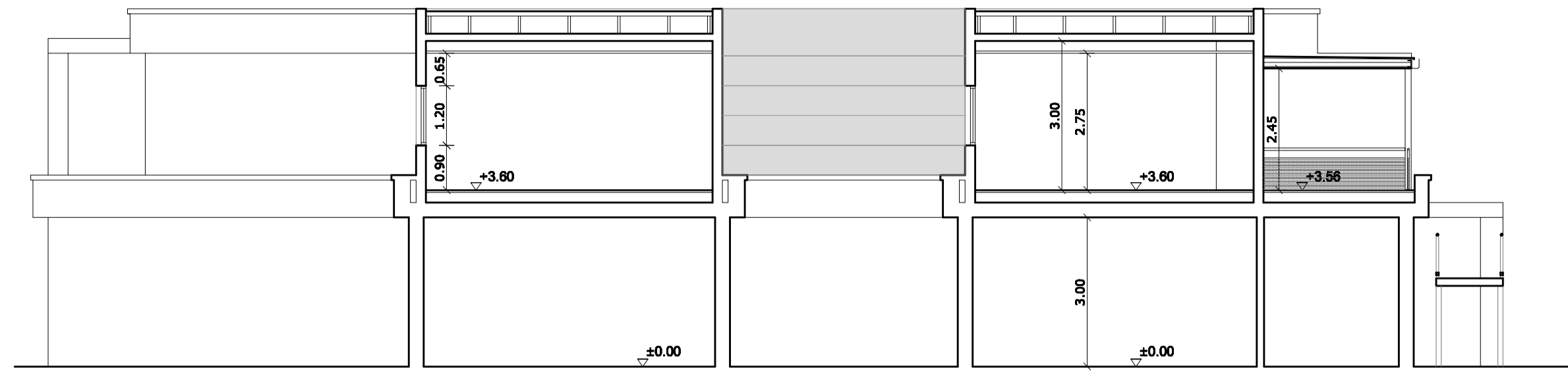
SECCION AA. ESTADO REFORMADO
