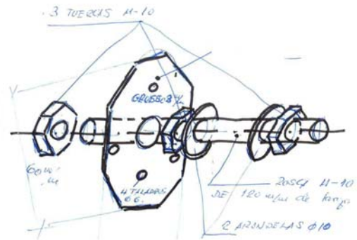
Zapata con pletina y tornillo roscado con tuercas auto-bloqueantes
